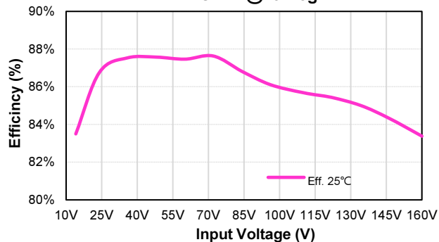
CQB50W12-72S12 Eff Vs Vin @25 Deg. C
