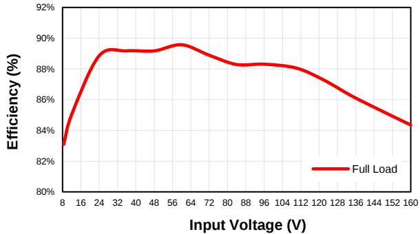
EC7BW18-72S15 Eff Vs Vin @25 Deg. C
