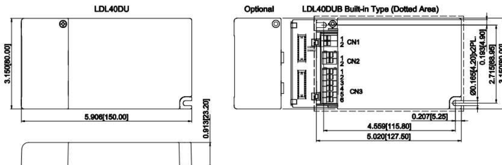
CN1:
